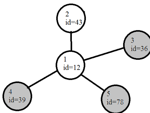
Рисунок 3.2 – Результат работы алгоритма (1-5 этапы)
