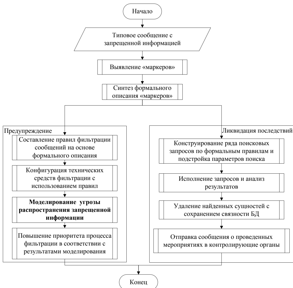
Рисунок 4.24 – Алгоритм противодействия распространению угрозы запрещенной информации
