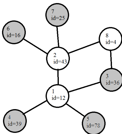
Рисунок 3.4 – Итоговый результат работы алгоритма
