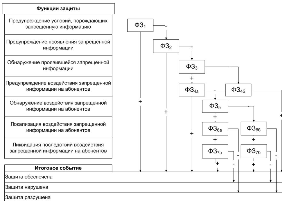
Рисунок 1.4 – Функции защиты от запрещенной информации в ИТКС
