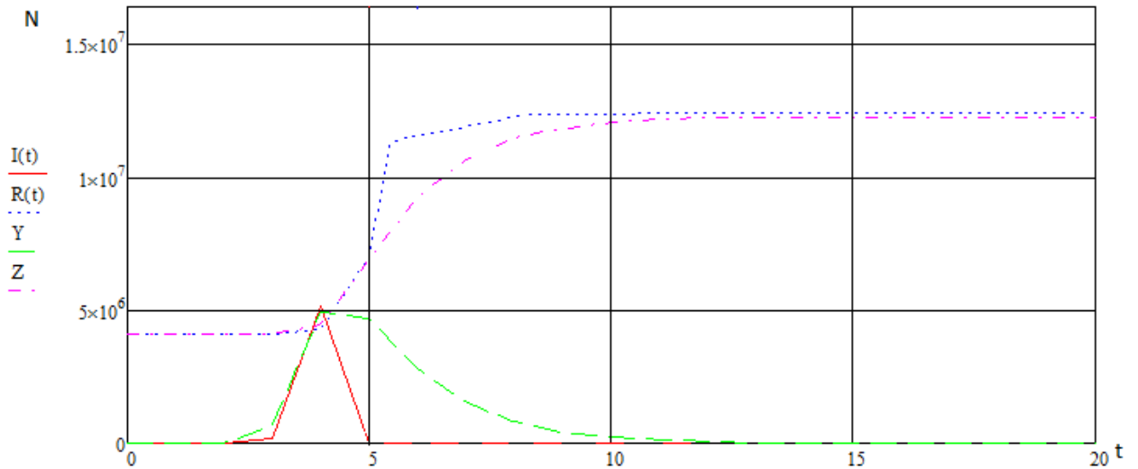
Рисунок 2.13 – Результаты аналитической и имитационной модели ( I и R – аналитическое решение, Y и Z – результаты имитационной модели). \beta=0,5 , \gamma=0,51 , R_0 \approx 4 \cdot 10^6 , I_0 = 1 .
