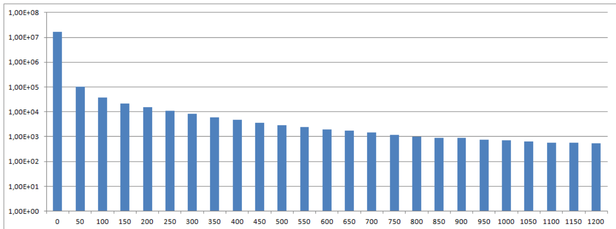
Рисунок 4.16 – Распределение степеней связности по всем узлам (ВКонтакте)
