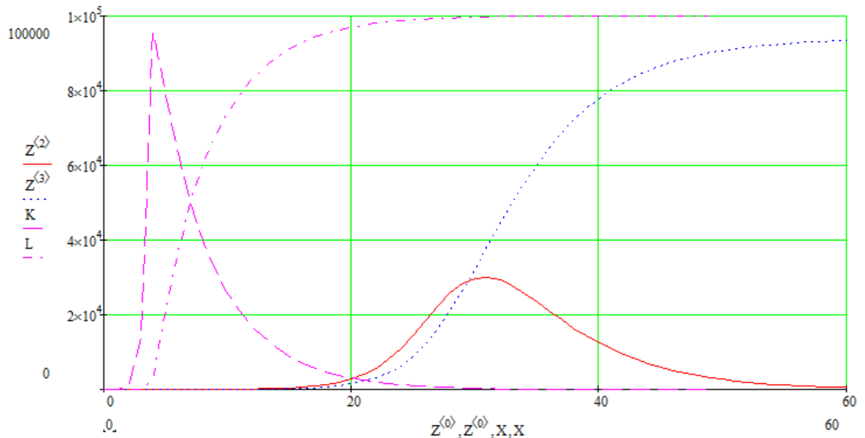
Рисунок 2.8 – Результаты имитационного моделирования ( N=100000 , \varphi = 150 , I_0=1 , \beta=0,3 , \gamma =0,2 , R_0=0 ) и аналитического решения ( Z^{<2>} , Z^{<3>} - аналитическое решение для процессов атаки и защиты соответственно, K , L – результаты имитационного моделирования для процессов атаки и защиты соответственно)
