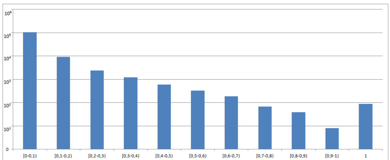
Рисунок 4.22 – Распределение кластерного коэффициента (ВКонтакте)
