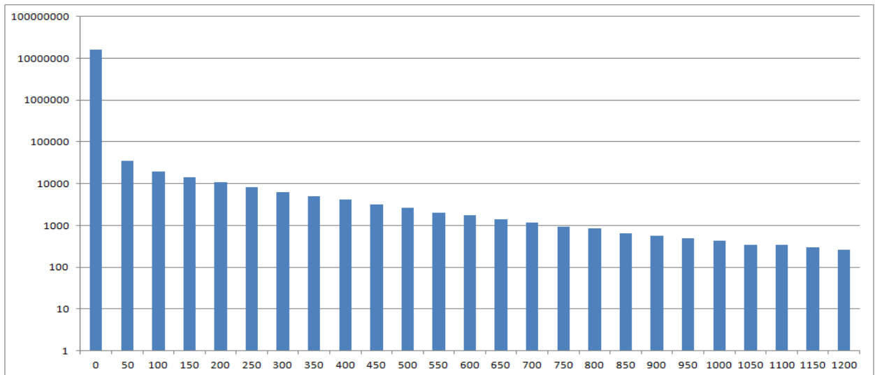
Рисунок 4.19 – Распределение степеней связности по всем узлам (Facebook)
