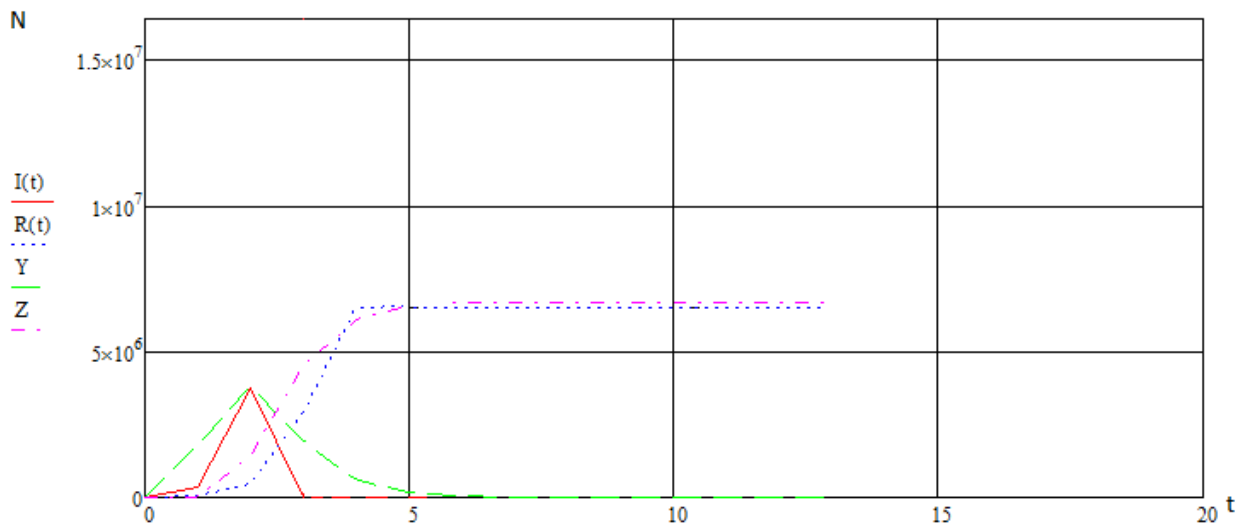
Рисунок 2.12 – Результаты аналитической и имитационной модели ( I и R – аналитическое решение, Y и Z – результаты имитационной модели). \beta=0,5 , \gamma=0,51 , R_0=0 , I_0 \approx 24000 .
