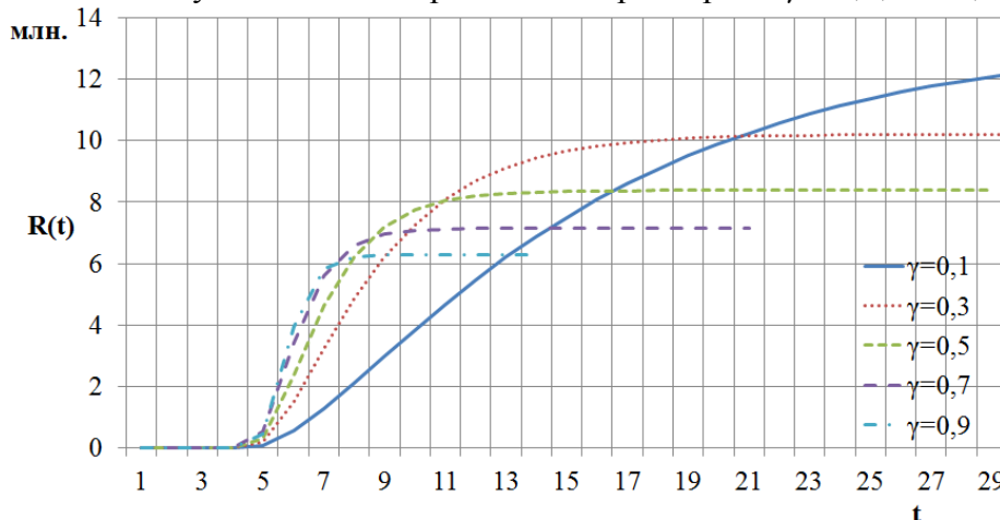
Рисунок 4.2 – Результаты моделирования с параметрами \beta = 0,2 , I_0 = 1 , R_0 = 0
