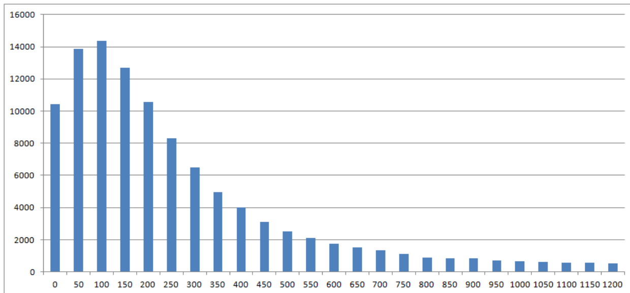
Рисунок 4.17 - Распределение степеней связности по открытым узлам (ВКонтakte)
