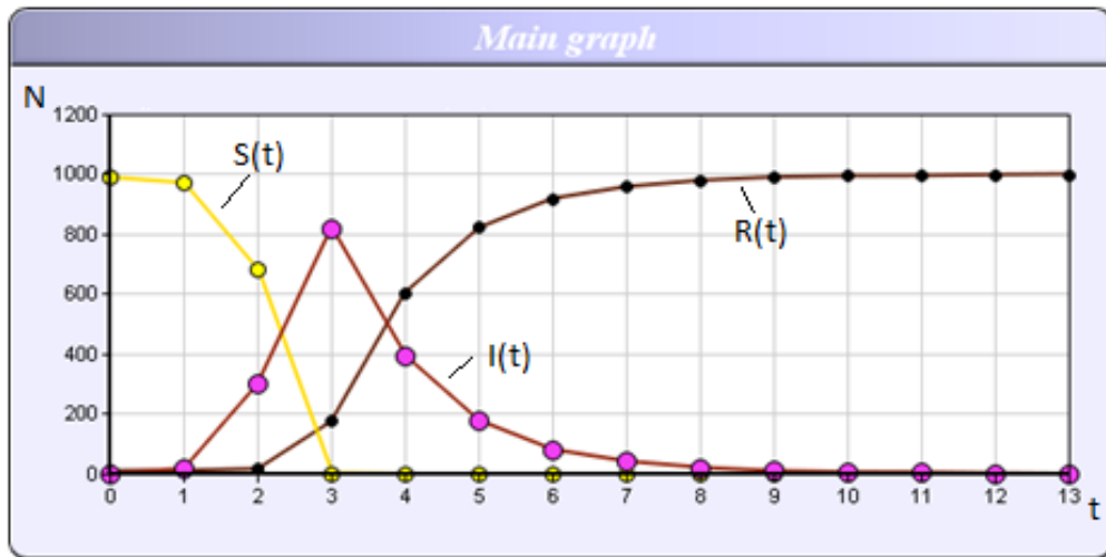
Рисунок 2.7 – Имитационное моделирование ( N=1000 , \varphi = 20 , I_0=1 , \beta=0,5 , \gamma =0,5 , R_0 =10 ), S(t) – количество подверженных атаке узлов
