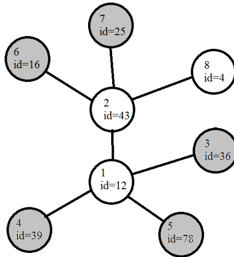
Рисунок 3.3 – Результат работы алгоритма (1-9 этапы)
