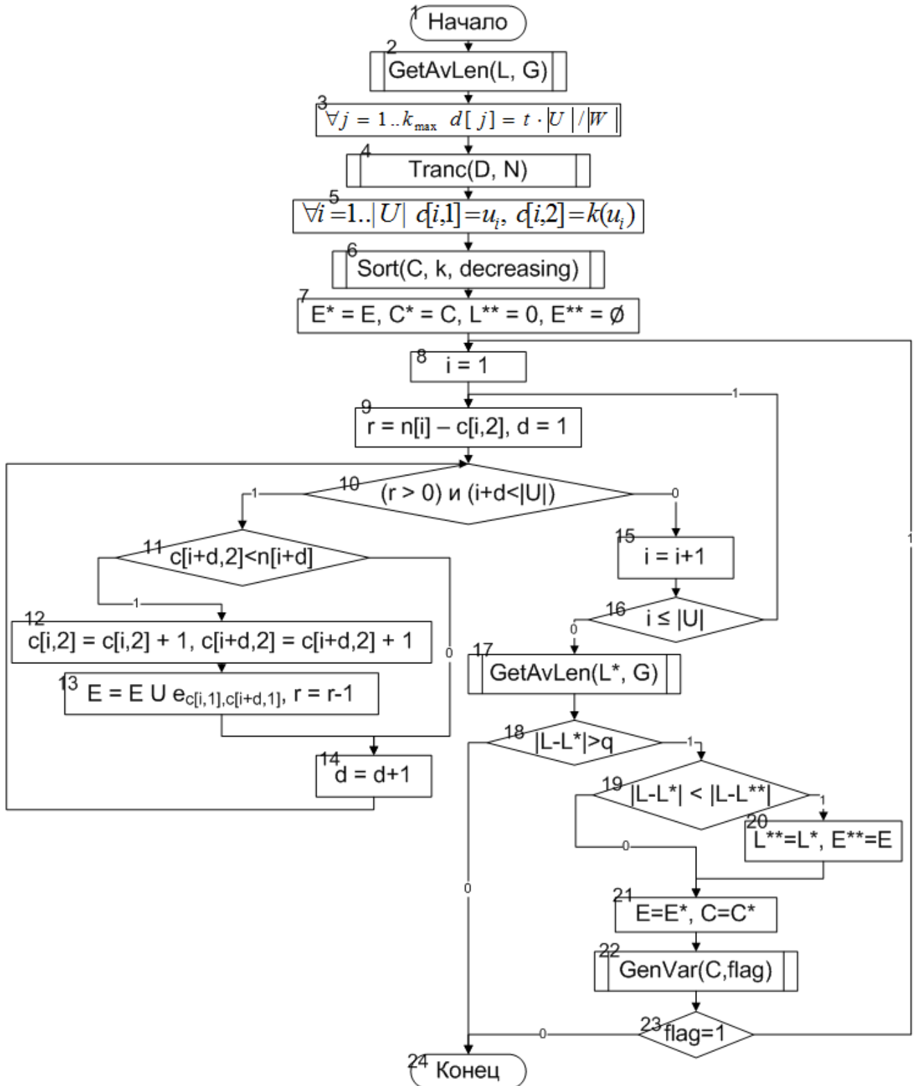
Рисунок 3.6 – Алгоритм генерации недоступной части сети
