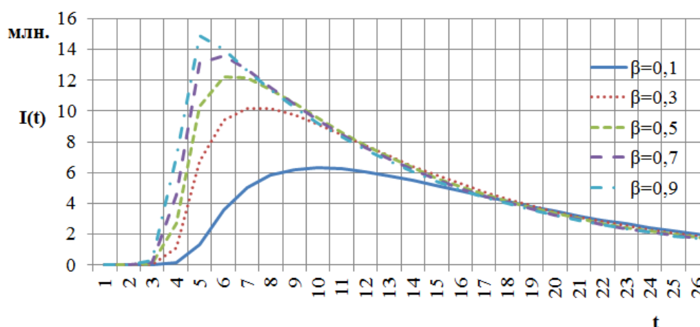
Рисунок 4.1 – Результаты моделирования с параметрами \gamma = 0,1 , I_0 = 1 , R_0 = 0
