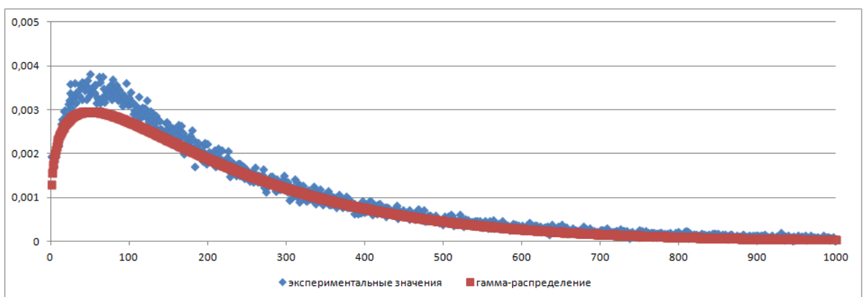
Рисунок 4.21 – Экспериментальное и аппроксимирующее распределения средней степени связности (Facebook)
