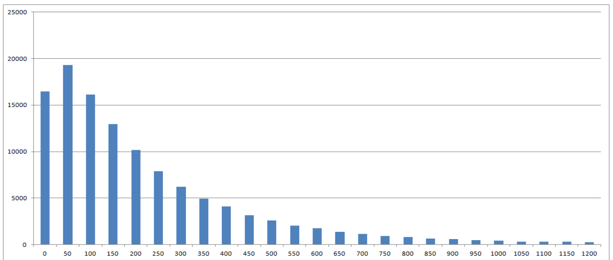
Рисунок 4.20 - Распределение степеней связности по открытым узлам (Facebook)
