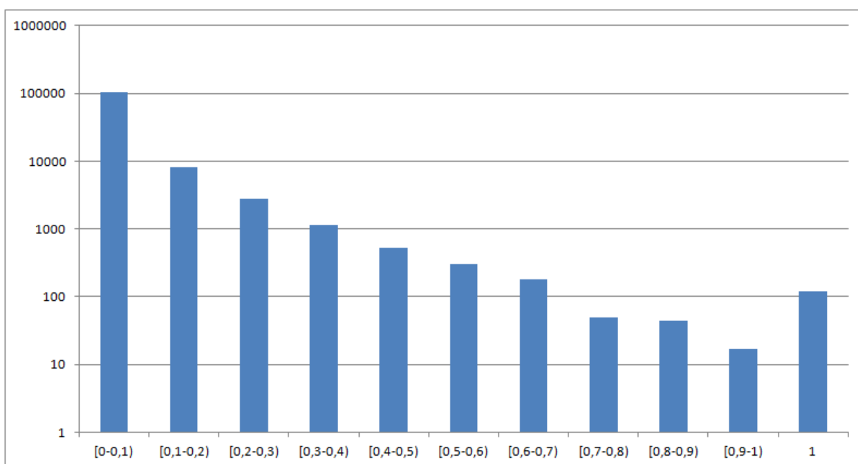
Рисунок 4.23 – Распределение кластерного коэффициента (Facebook)
