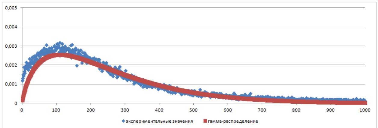
Рисунок 4.18 – Экспериментальное и аппроксимирующее распределения средней степени связности (ВКонтакте)
