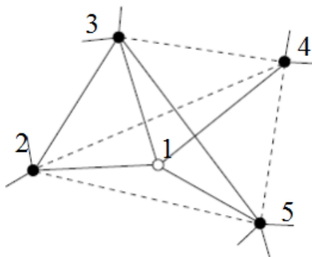
Рисунок 3.5 – Схематичный рисунок для определения кластерного коэффициента
