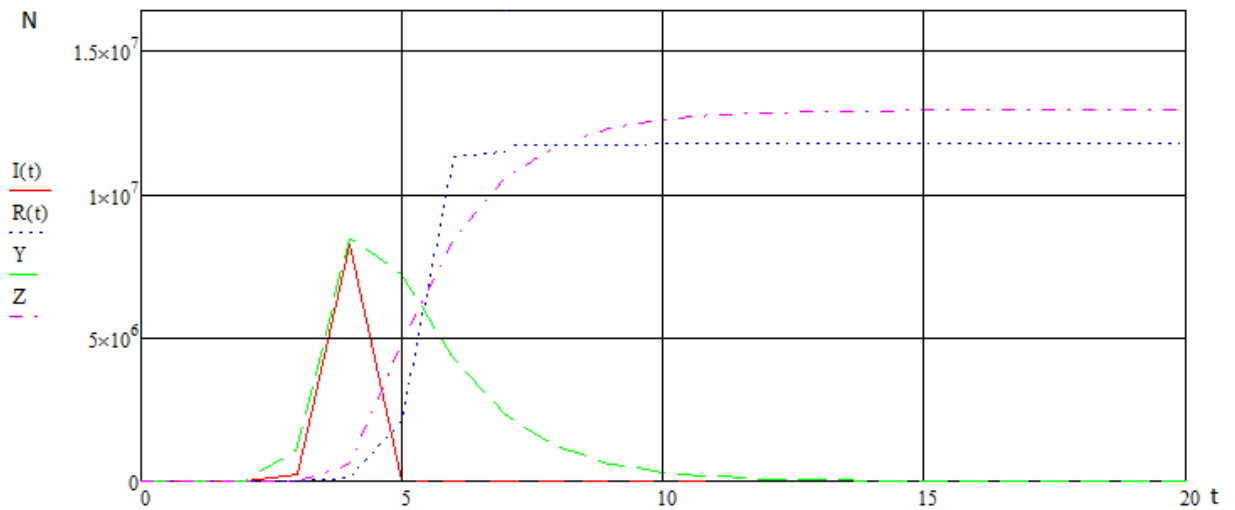
Рисунок 2.11 – Результаты аналитической и имитационной модели ( I и R – аналитическое решение, Y и Z – результаты имитационной модели). \beta=0,5 , \gamma=0,51 , R_0=0 , I_0=1 .
