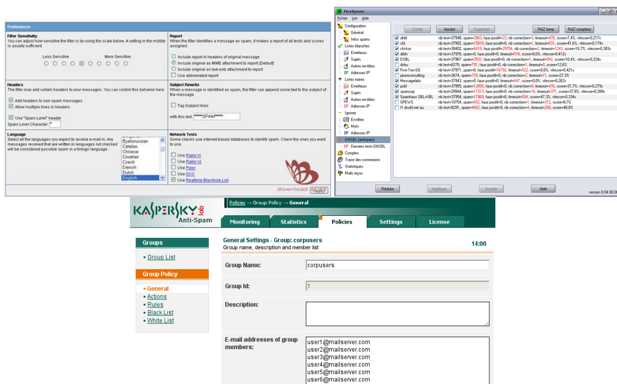
Рисунок 4.27 – Скриншоты программ
