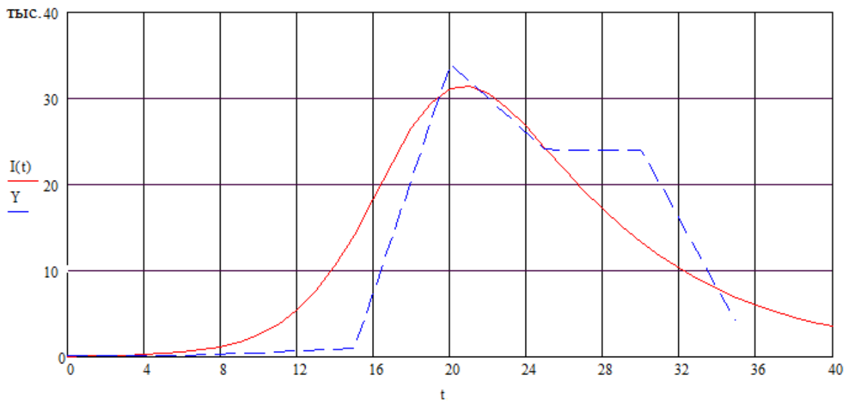
Рисунок 4.28 – Исходные данные (Y) и результат аналитической модели (I), условная единица времени равна 5 часам
