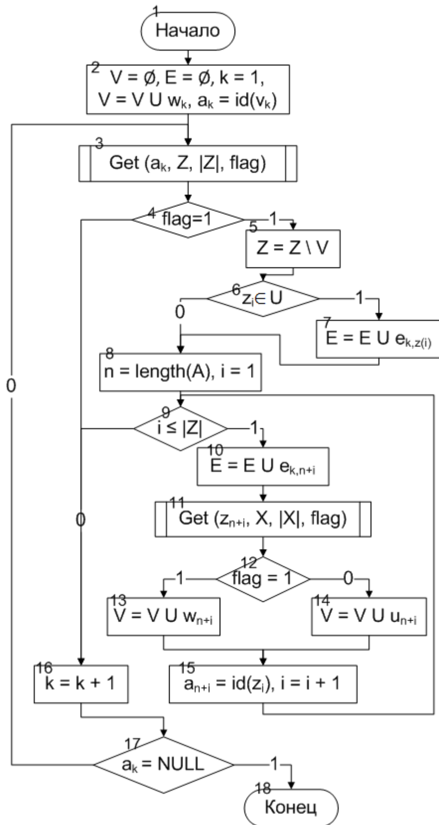
Рисунок 3.1 – Блок-схема алгоритма формирования графа доступной части сети
