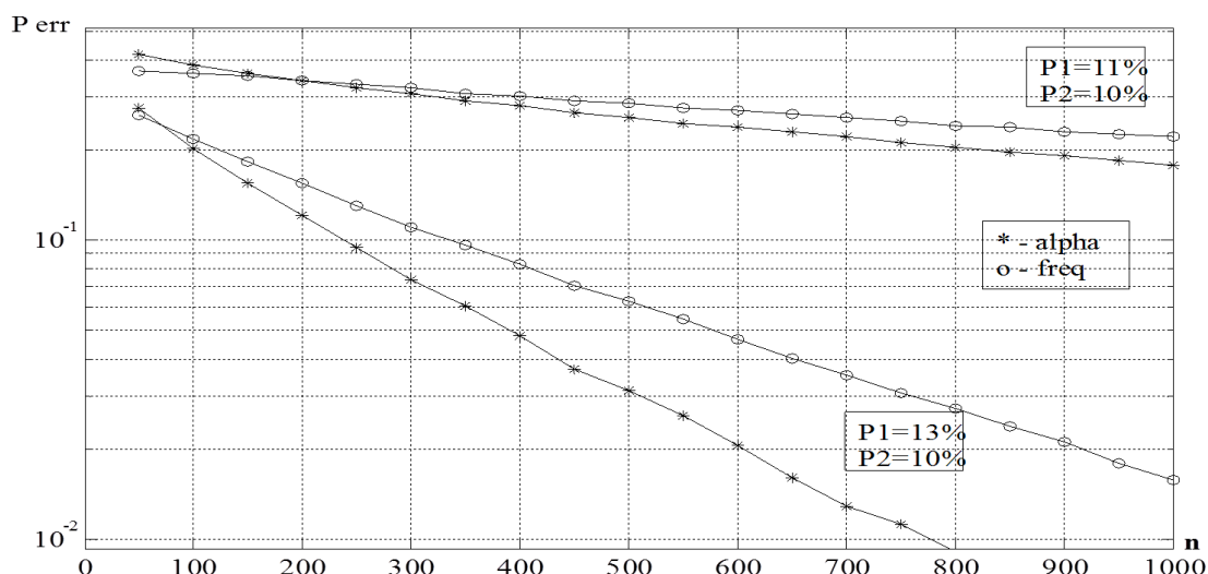
Рисунок 2. Зависимость вероятности ошибочного решения при сравнении САГК от объема тестовой выборки звукозаписей
