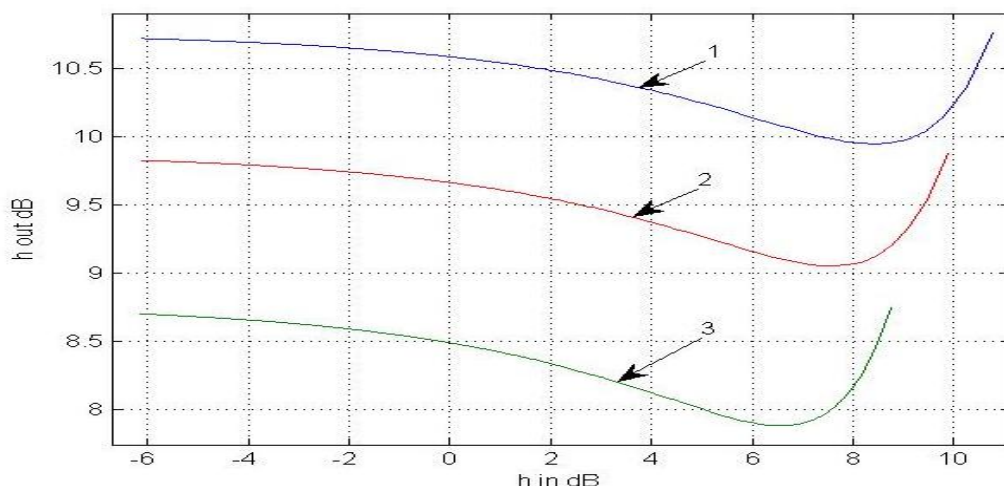
Рисунок 4. Графики зависимости отношения сигнал-шум на выходе компенсатора от отношения сигнал-шум на его входе
